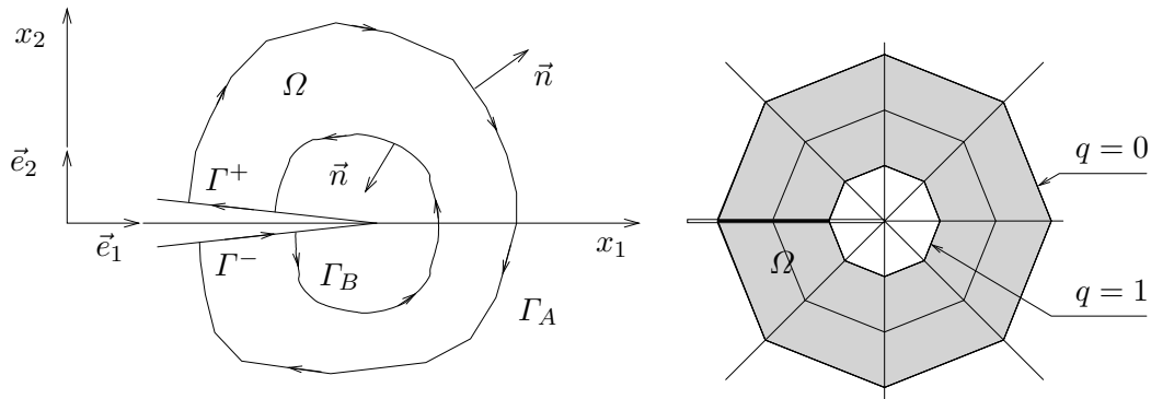
Fig. 11.13 : J-integral domain.
